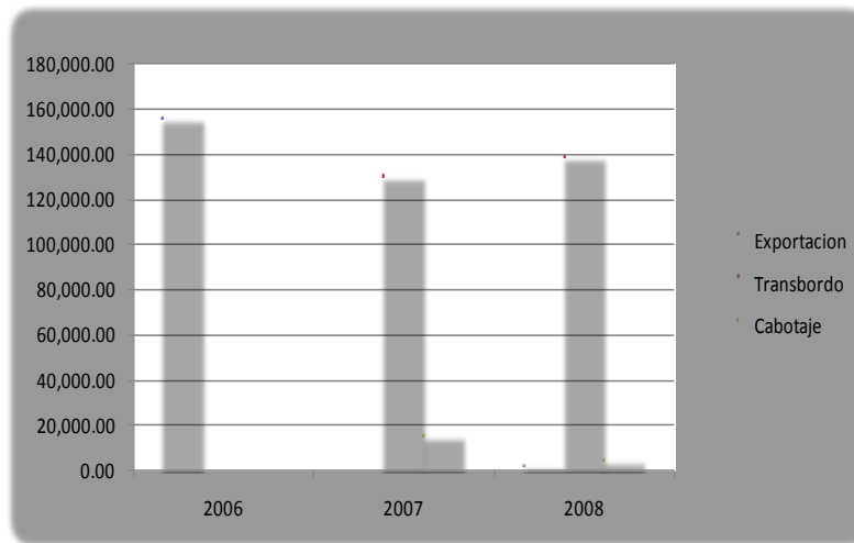
Gráfico 21: Terminal Portuario de Líquidos Tramarsa S.A. Movimiento de granel líquido (2006 - 2008) (Toneladas métricas)
