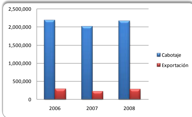
Gráfico 8: Terminal Portuario de Muelle Talara (Petroperú). Carga granel líquido (2006 - 2008) (Toneladas métricas)
