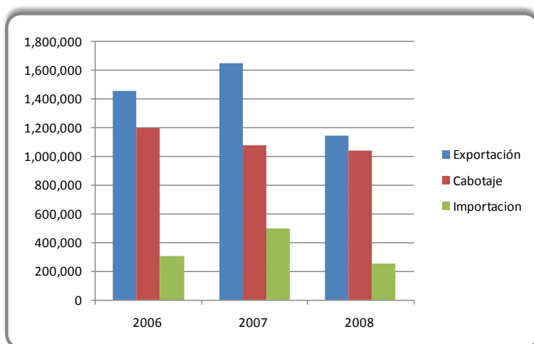
Gráfico 37: Terminal Portuario Bayovar (Petroperú). Movimiento de granel sólido (2006 - 2008) (Toneladas métricas)
