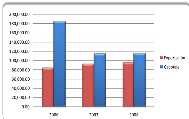
Gráfico 30: Terminal Portuario Terminal de Paramonga (Quimpac). Movimiento de granel líquido (2006 - 2008) (Toneladas métricas)
