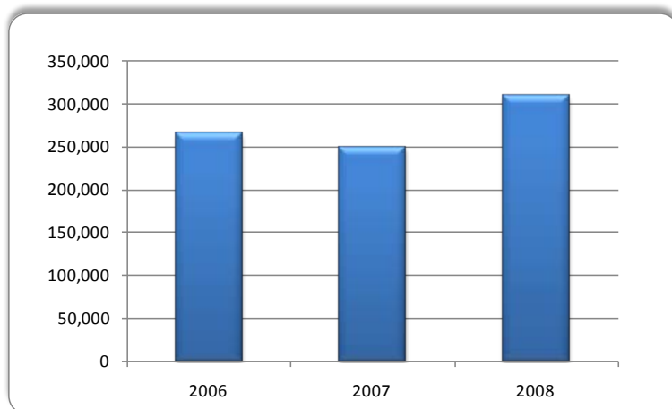
Gráfico 13: Terminal Portuario Amarradero Chimbote (Consortio Terminales). Movimiento de Granel Líquido (2006 - 2008) (Toneladas métricas)
