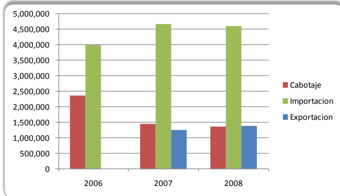
Gráfico 15: Terminal Marítimo Refinería La Pampilla (Repsol YPF). Carga granel líquido (2006 - 2008) (Toneladas métricas)
