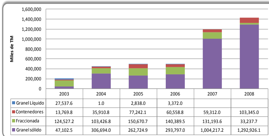
Gráfico 7: Terminal Portuario de Matarani. Movimiento de carga de exportación (2003 - 2008) (Toneladas métricas)
