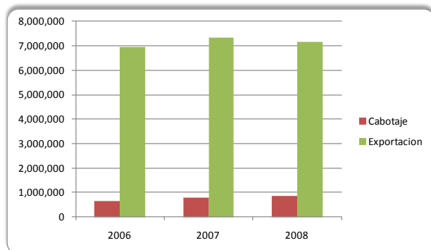
Gráfico 27: Terminal Portuario de San Nicolás. Carga a granel sólido (2006 - 2008) (Toneladas métricas)
