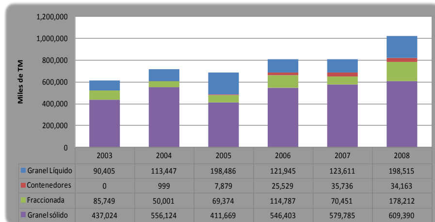
Gráfico 6: Terminal Portuario de Matarani. Movimiento de carga de importación (2003 - 2008) (Toneladas métricas)
