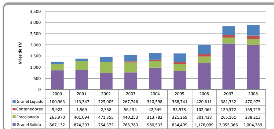
Gráfico 5: Terminal Portuario de Matarani. Movimiento de carga (2000 -2008) (Toneladas métricas)
